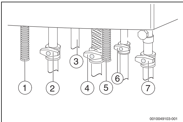
31. ábra Gáz- és vízdali csatlakozások (külön rendelhető tartozékok)
