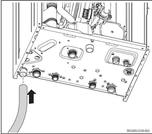
30. ábra A tömlő felszerelése a kondenzvíz szifonra
