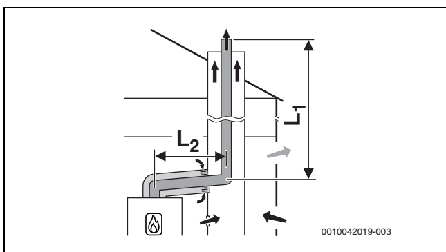
15. ábra B 53p szerinti merev füstgázvezetés aknában, környezeti levegőtől függő levegőellátással a felállítási helyiségben lévő koncentrikus összekötő vezetéken keresztül; hátsó szellőzőnyílás az aknában
